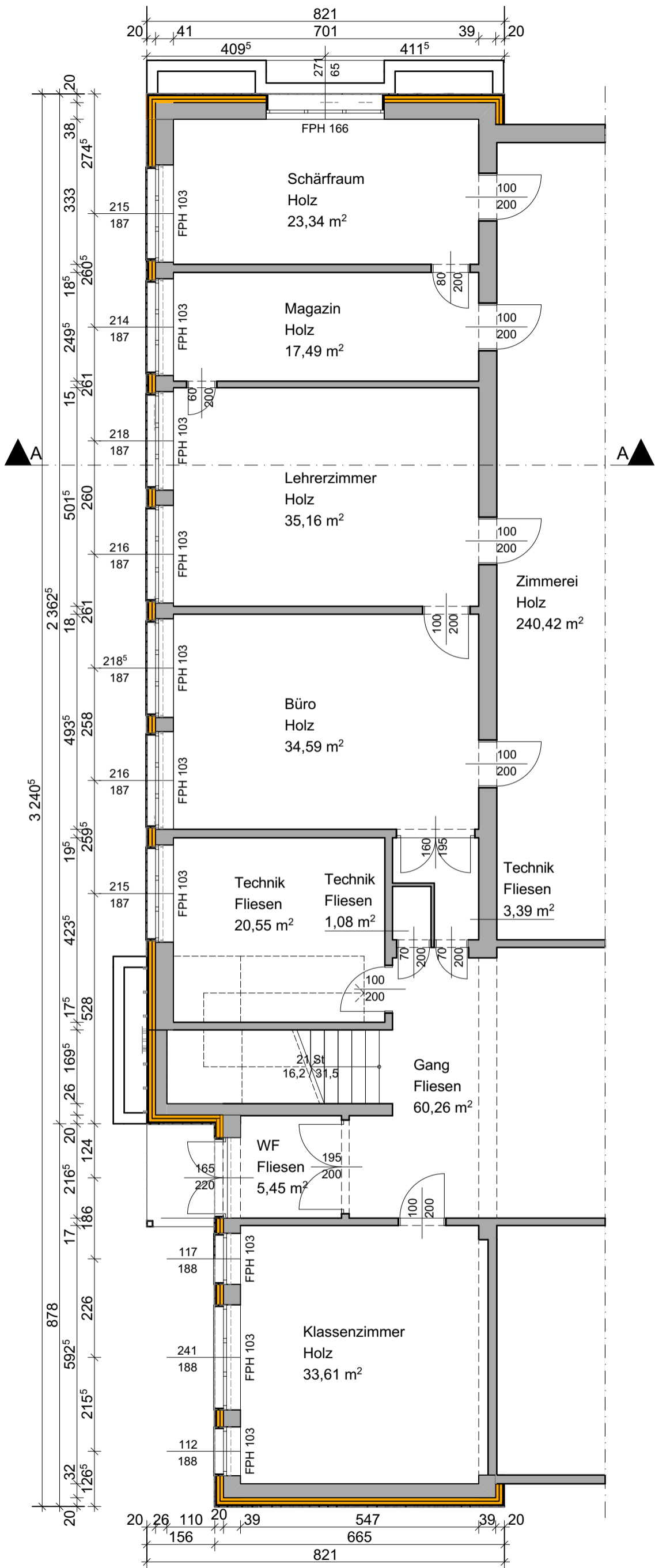
ERDGESCHOSS
