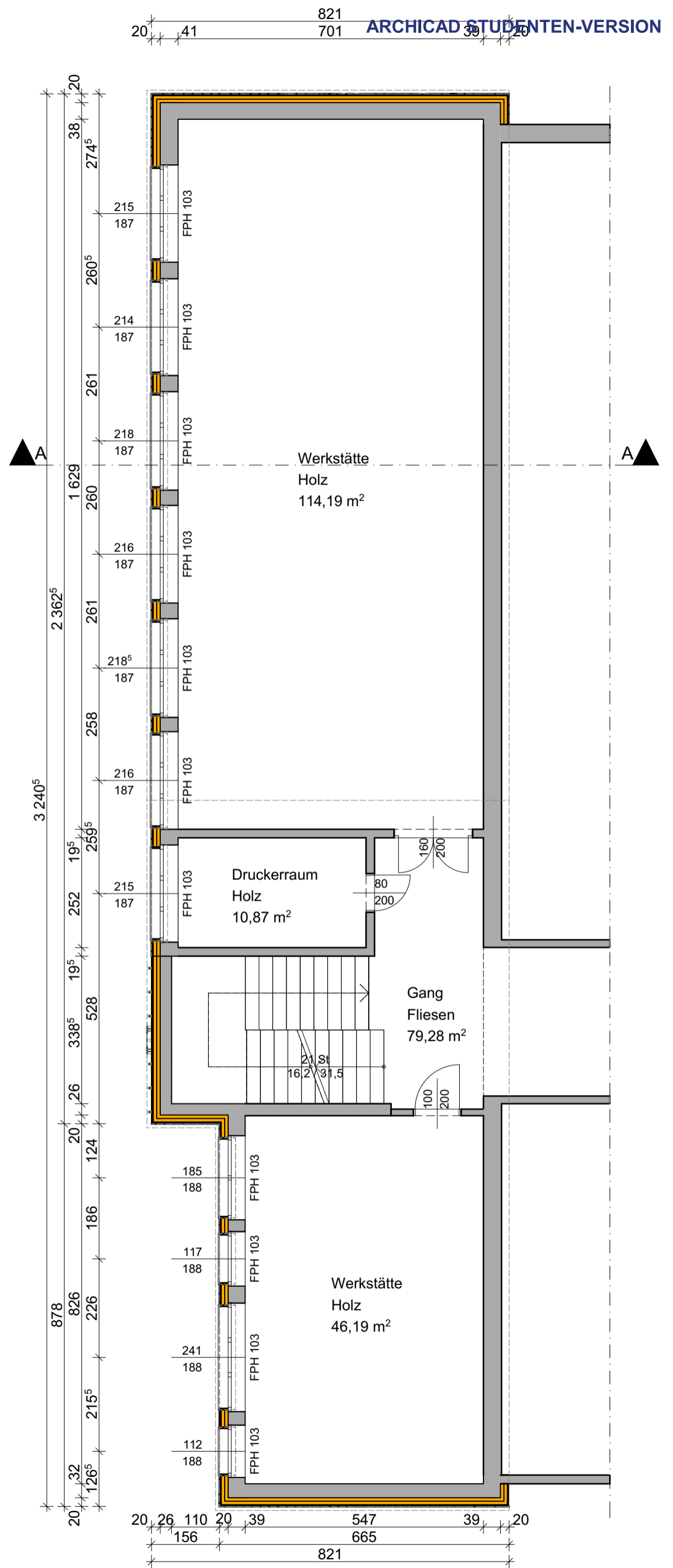
OBERGESCHOSS
